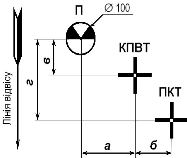
Контрольно-вивірочна мішень БТР-80
