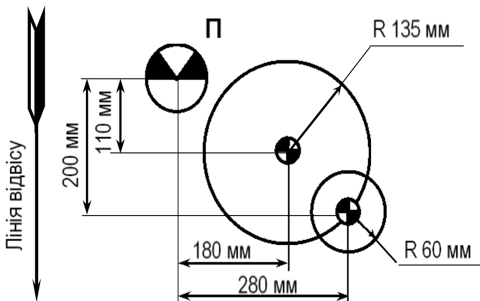
Пристрілочна мішень БТР-80
