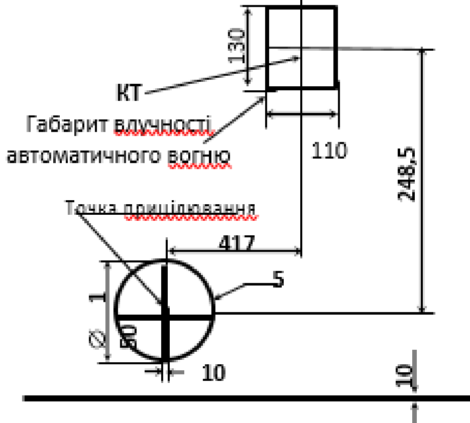
Пристрілочна мішень для спареного кулемету ПКТ БМП-1 (БРМ-1К)
